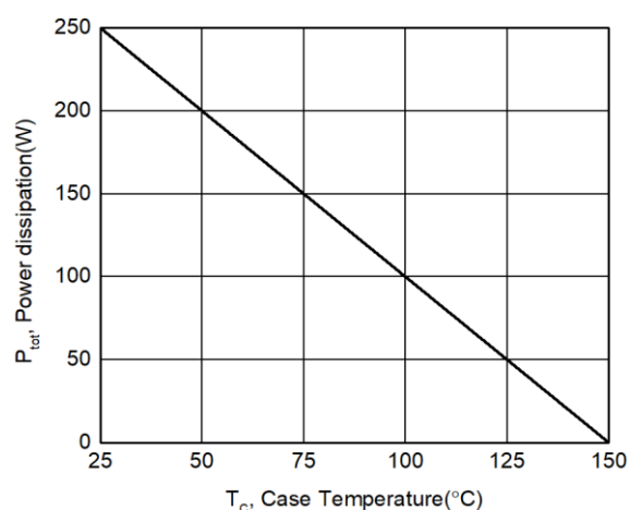
图 5 耗散功率与壳温的关系 ( T_j \leq 150^{\circ}\text{C} )
