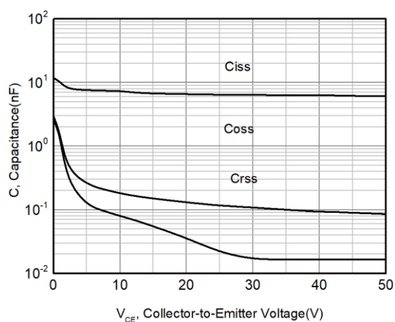
图 3 电容与集电极-发射极电压的关系 ( V_{GE}=0\text{V} , f=1\text{MHz} )
