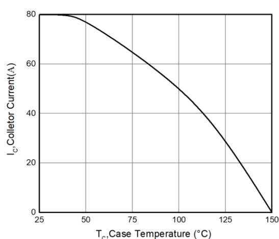
图 6 集电极电流与壳温的关系 ( V_{GE} \geq 15\text{V} , T_j \leq 150^{\circ}\text{C} )
