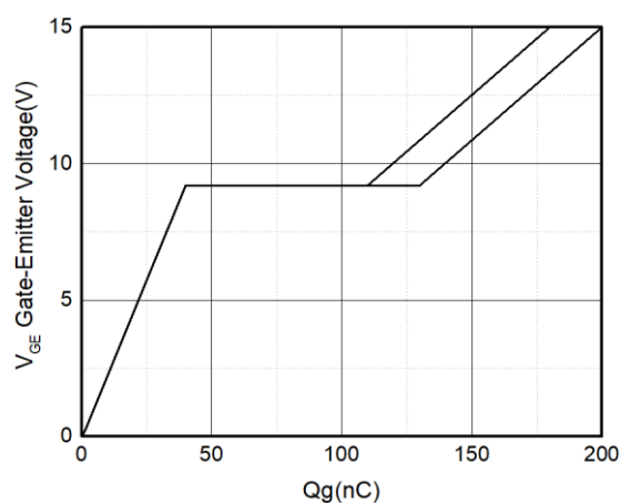
图 4 栅电荷特性 ( I_C=50\text{A} )
