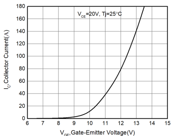
图 2 转移特性 ( V_{CE}=20\text{V} )
