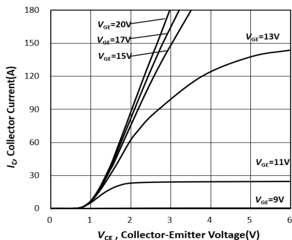
图 1 常温输出特性( T_j=25^{\circ}\text{C} )
