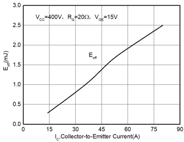
图7 关断损耗与集电极电流的关系 ( T_j \leq 150^\circ \text{C} )
