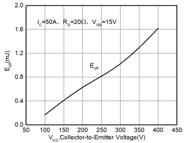
图8 关断损耗与集电极电压的关系 ( T_j \leq 150^\circ \text{C} )
