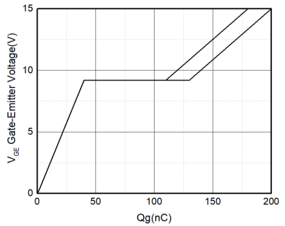
图4 栅电荷特性 ( I_C=50\text{A} )
