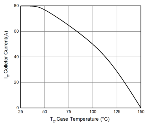
图6 集电极电流与壳温的关系 ( V_{GE} \geq 15\text{V}, T_j \leq 150^\circ\text{C} )
