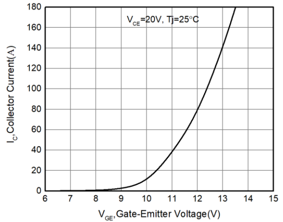
图2 转移特性 ( V_{CE}=20\text{V} )
