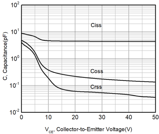
图3 电容与集电极-发射极电压的关系 ( V_{GE}=0\text{V}, f=1\text{MHz} )
